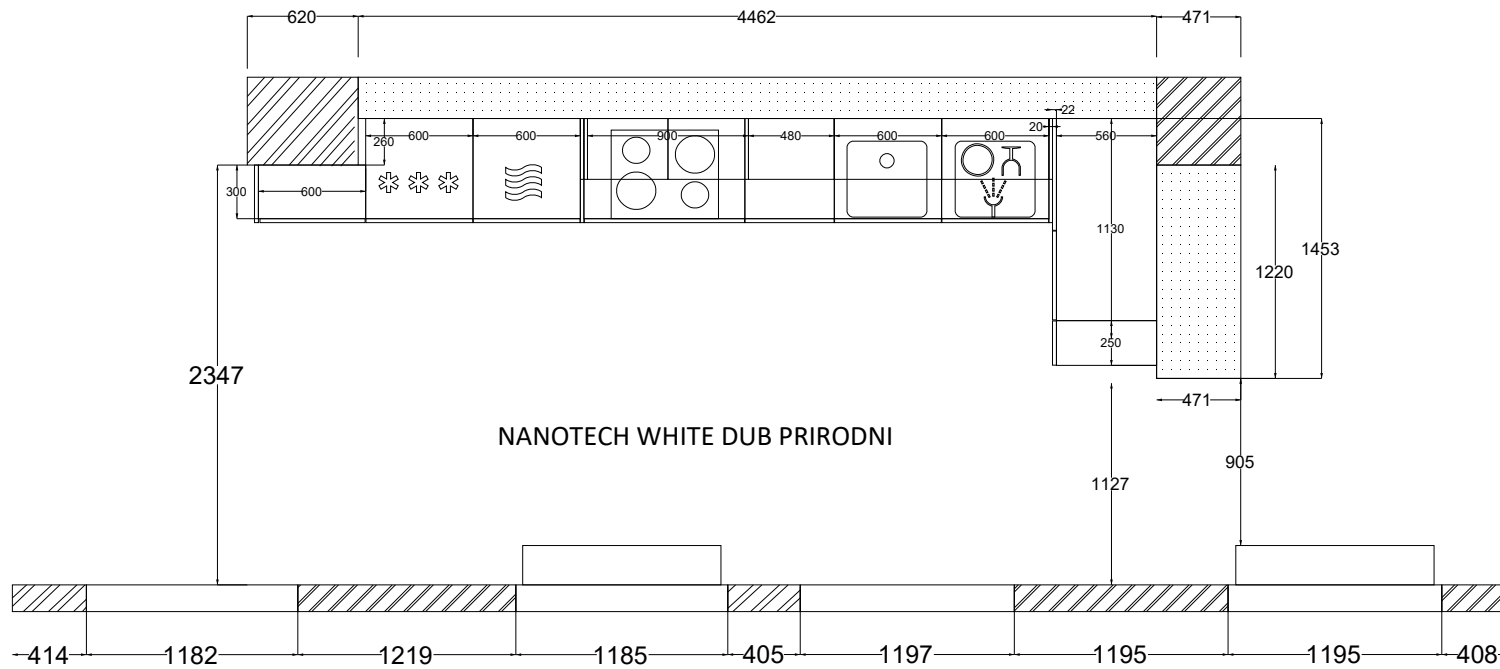
PŮDORYS
