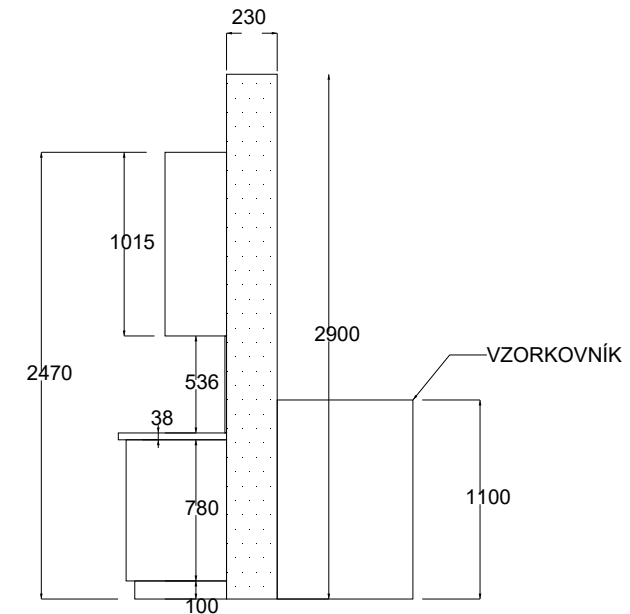
VÝŠKOVÉ KÓTY
